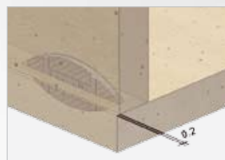
Dubbele groef voor Clamex
